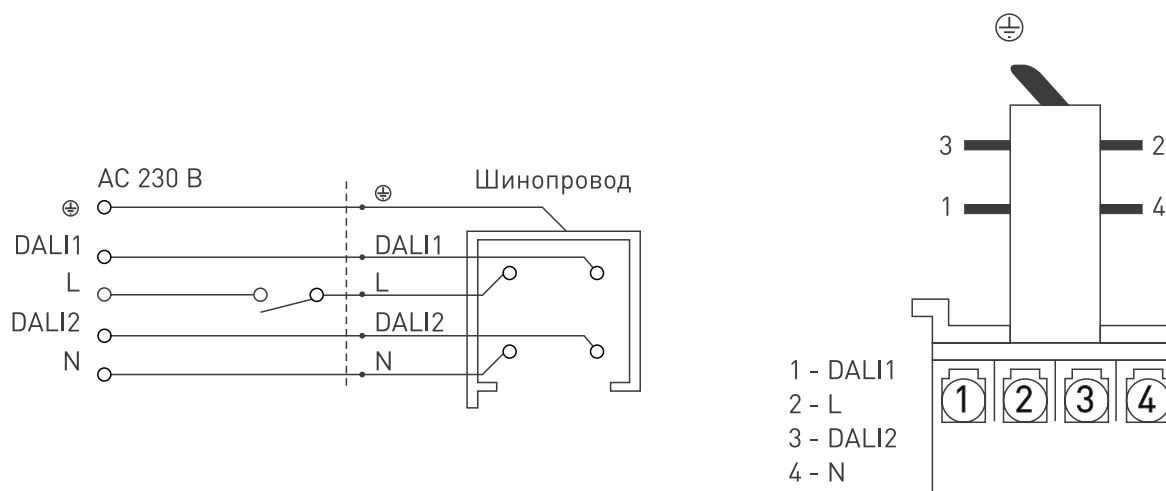
Рис. 2. Схема подключения
