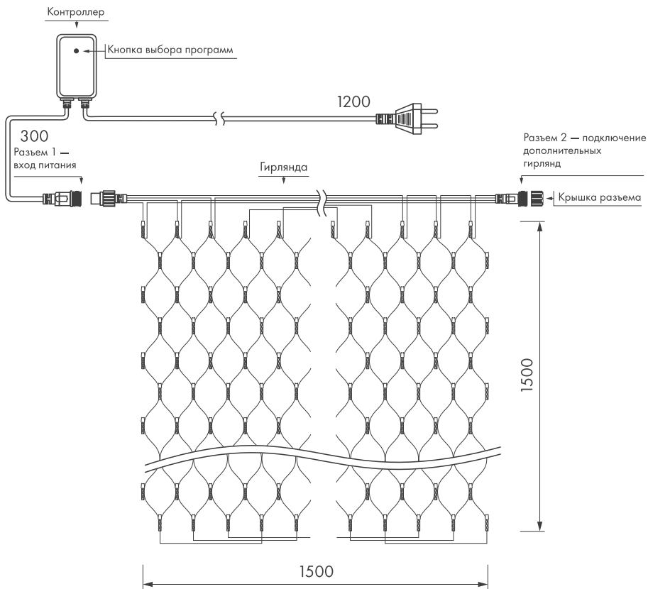
Рисунок 1. Схемы подключения
